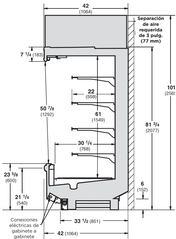
Corte transversal del CF5X
