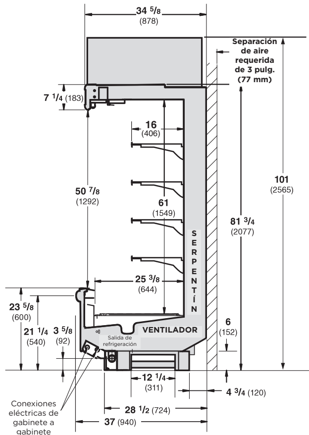
Corte transversal del DF5NX
