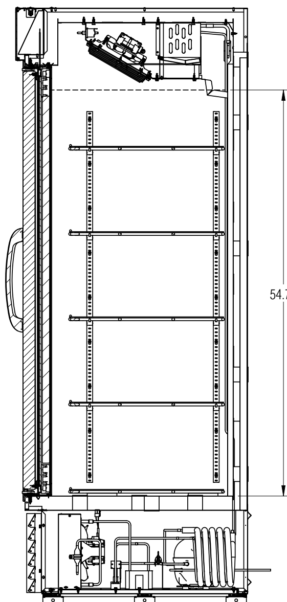
SECCIÓN A-A
