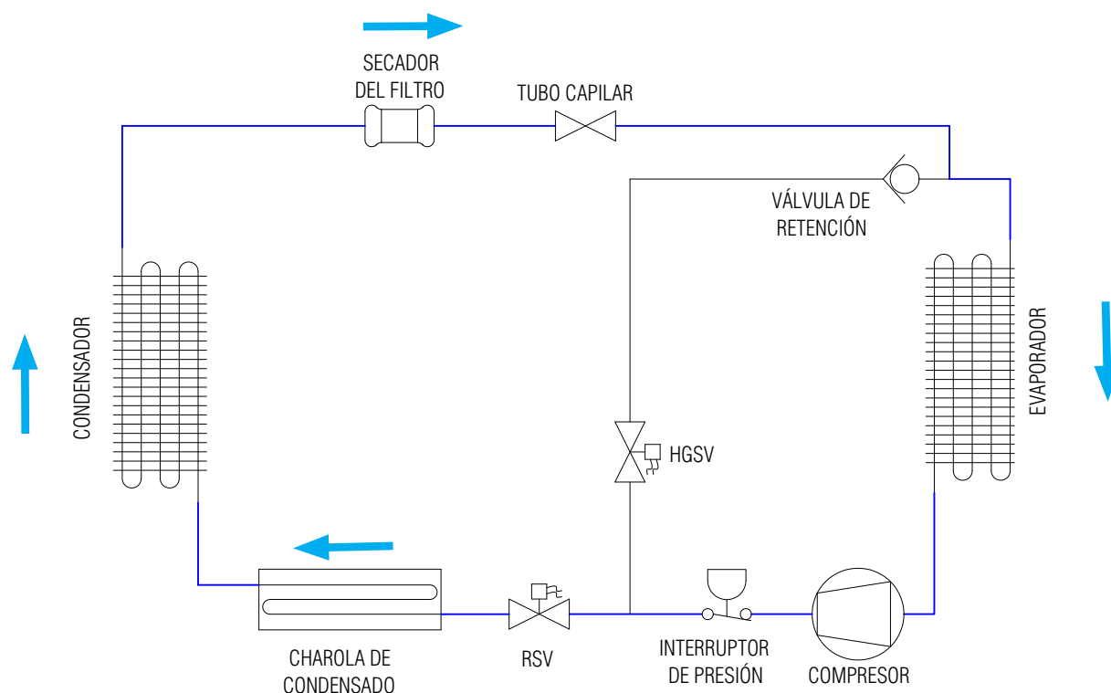
Figura A. Diagrama del sistema— Modo de refrigeración (Este diagrama se aplica a los modelos de 1 y 2 puertas)
