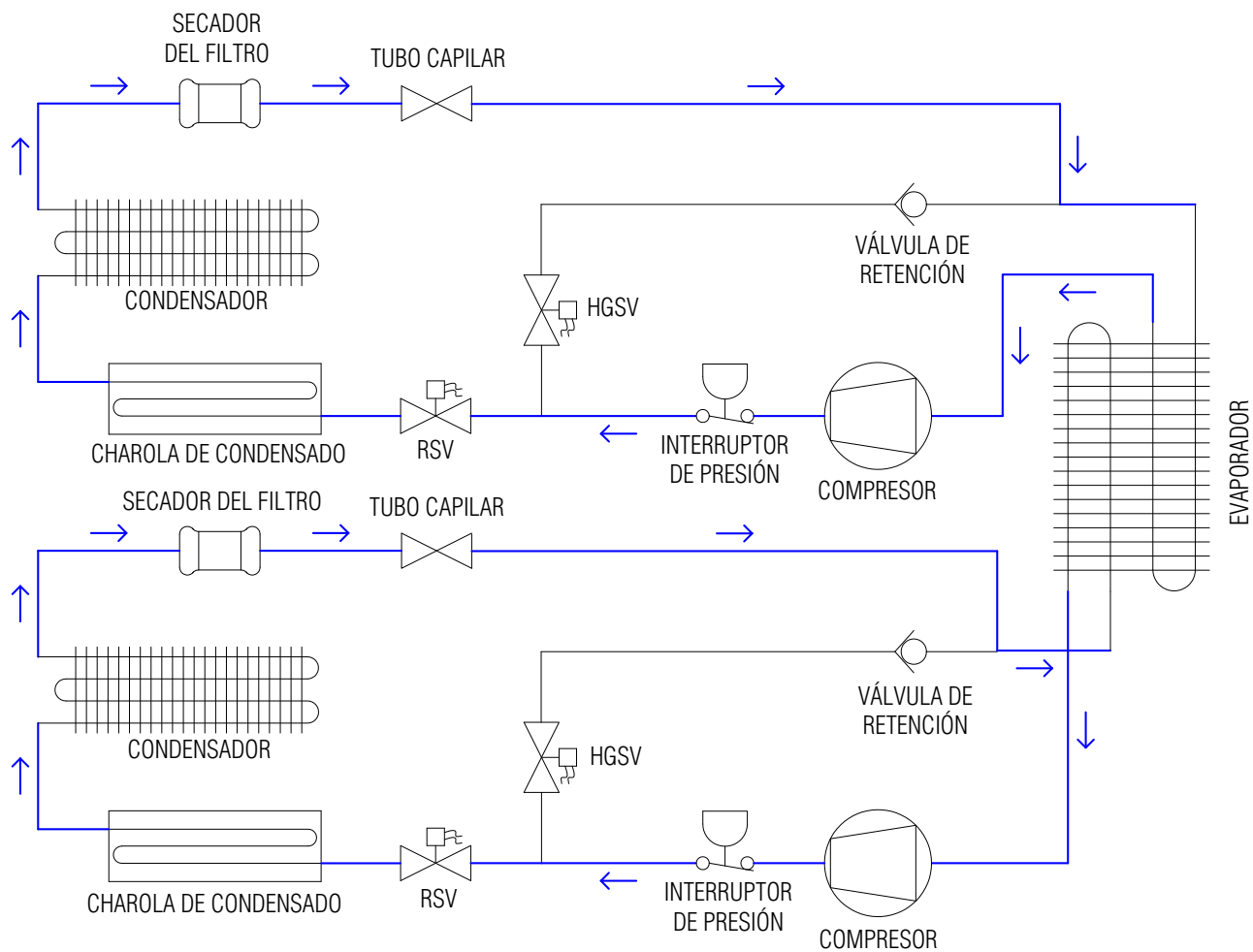
Figura A. Diagrama del sistema— Modo de refrigeración (Este diagrama se aplica a los modelos de 3 puertas)
