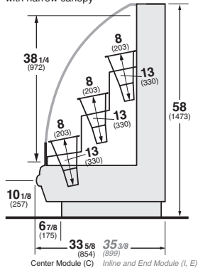
IM-CS-R Center Module / IM-IS-R In-Line Module
