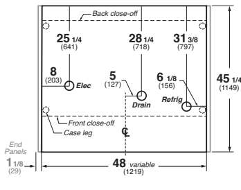
Q1-FC/FS Single-Deck Fish
