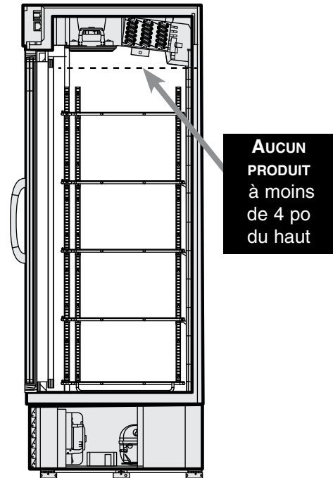
Limite de charge pour les comptoirs réfrigérés VRM
