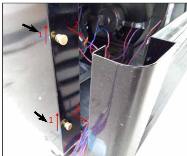
Desserrer les vis de chaque côté de la grille inférieure.
