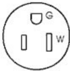
NEMA 5-15R
