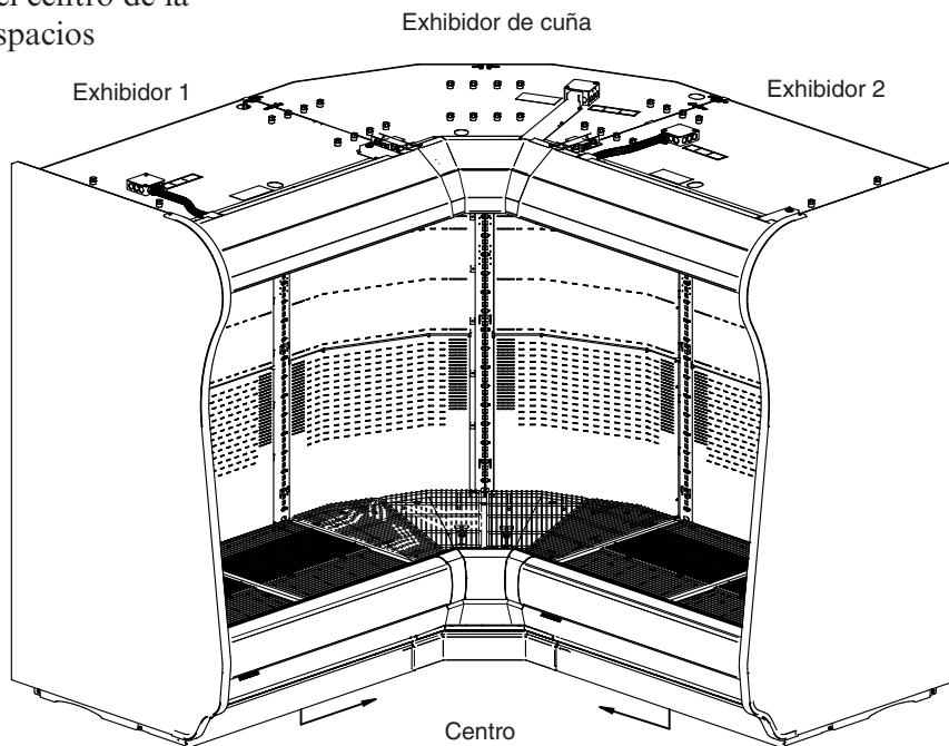
Alineación de exhibidores de cuña interior
