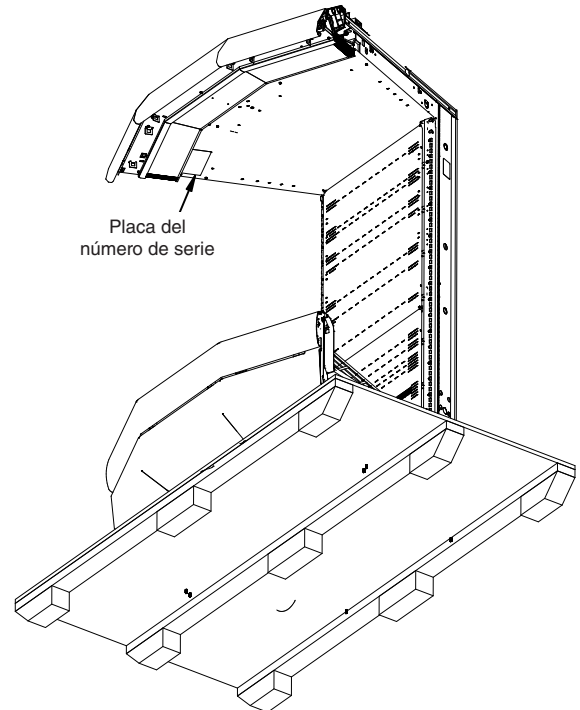
Placa con el número de serie ubicada dentro del toldo del exhibidor de cuña
