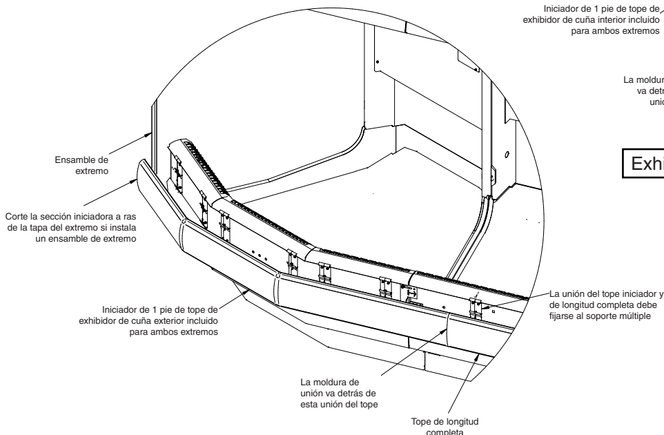
Exhibidor de cuña exterior
