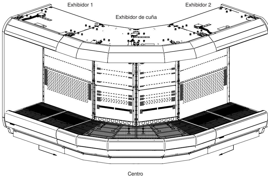
Alineación de exhibidores de cuña exterior
