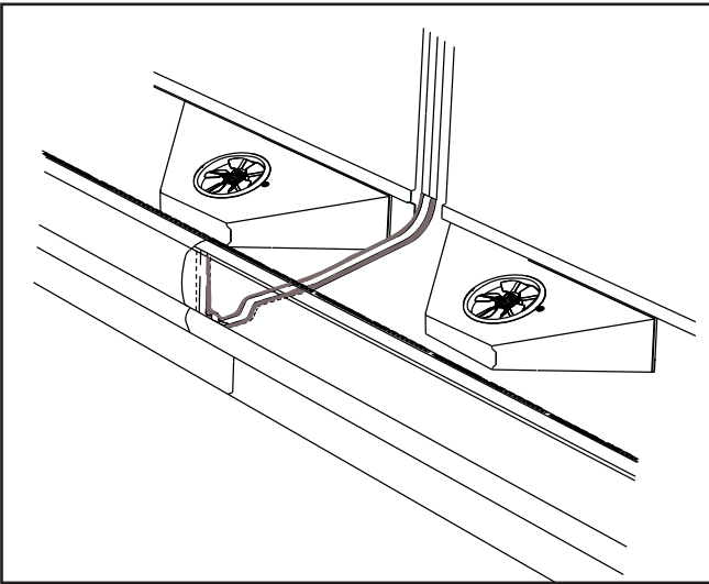
Aplique cinta de butilo - Exhibidor de cuña interior
