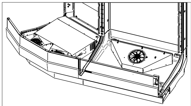
Aplique sellador de silicona de curado neutro Exhibidor de cuña exterior
