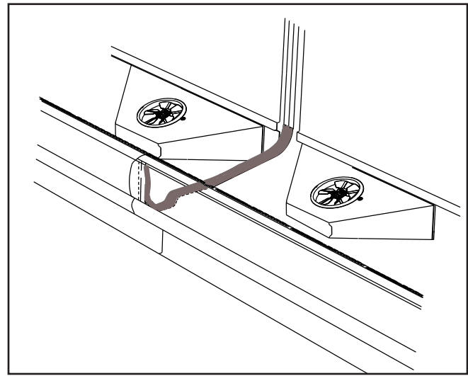
Aplique sellador de silicona de curado neutro Exhibidor de cuña interior
