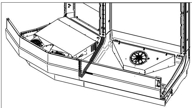
Aplique cinta de butilo - Exhibidor de cuña exterior
