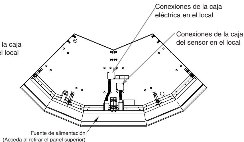
Exhibidor de cuña exterior de 90°
