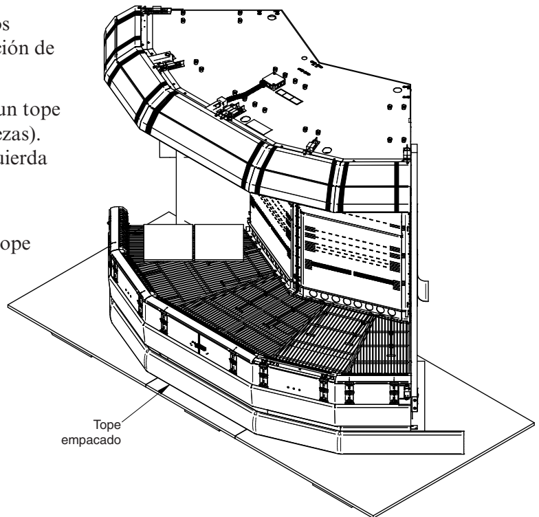
Exhibidor de cuña exterior
