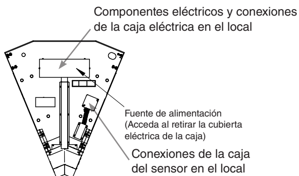
Exhibidor de cuña exterior de 45°
