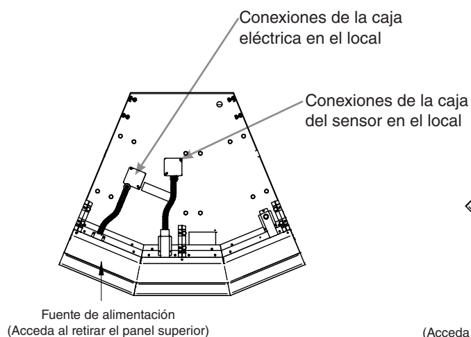
Exhibidor de cuña exterior de 45°
